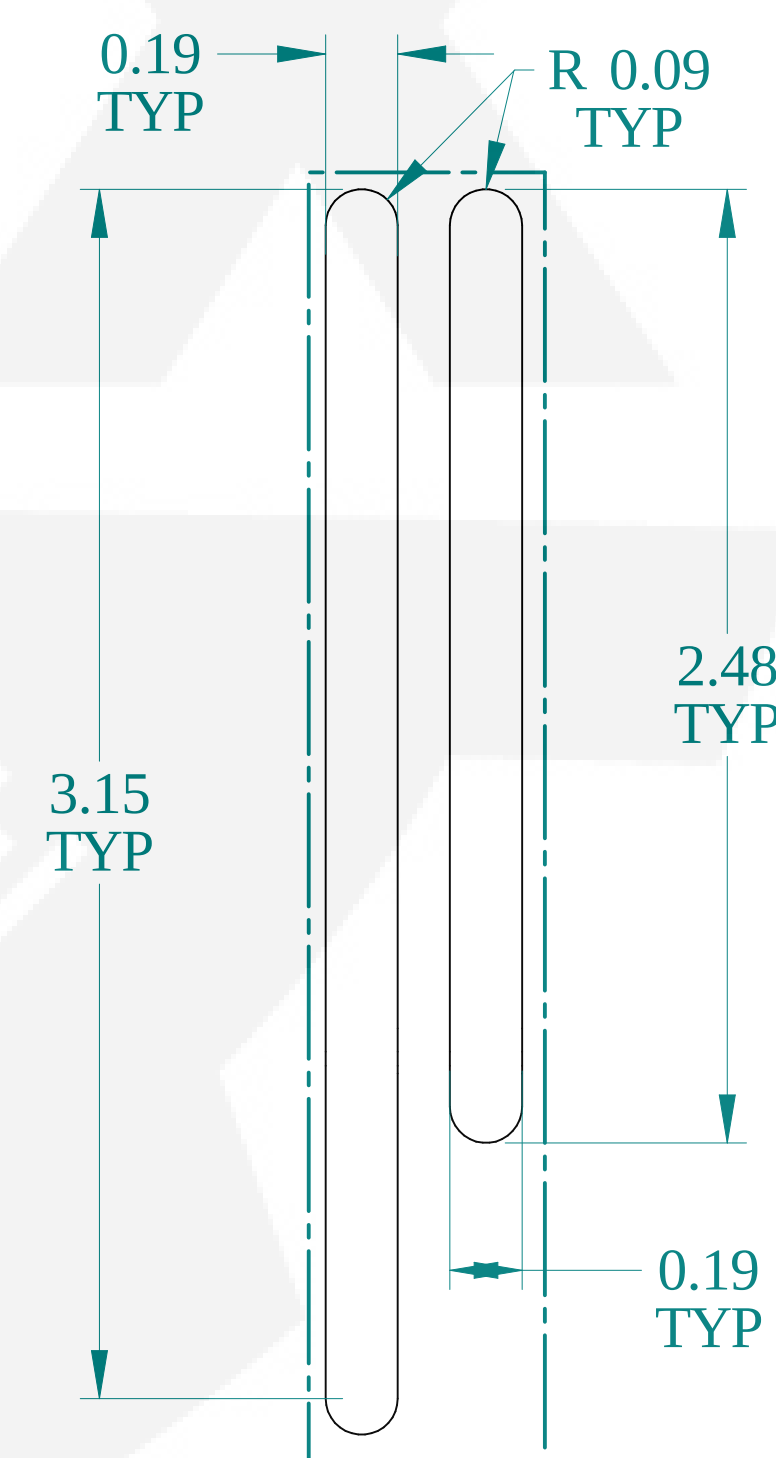
DETAIL Z TYP
