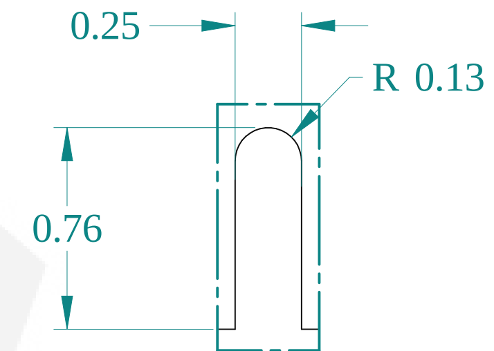
DETAIL Y TYP
