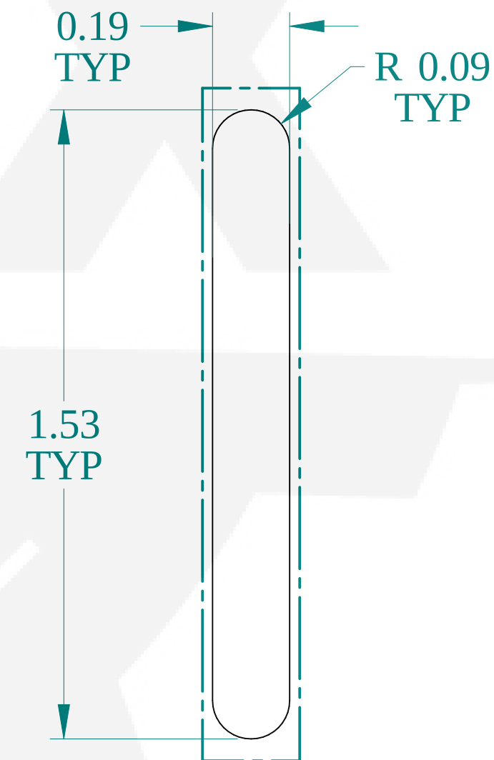
DETAIL Z TYP
