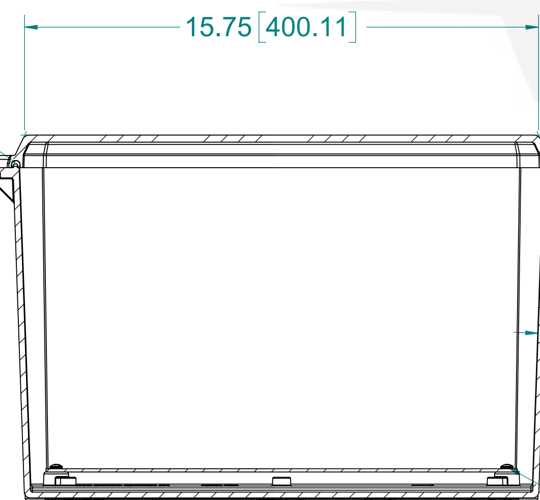
SECTION A-A
