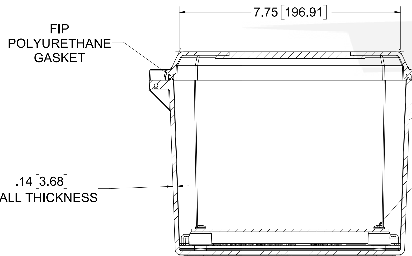
SECTION A-A
