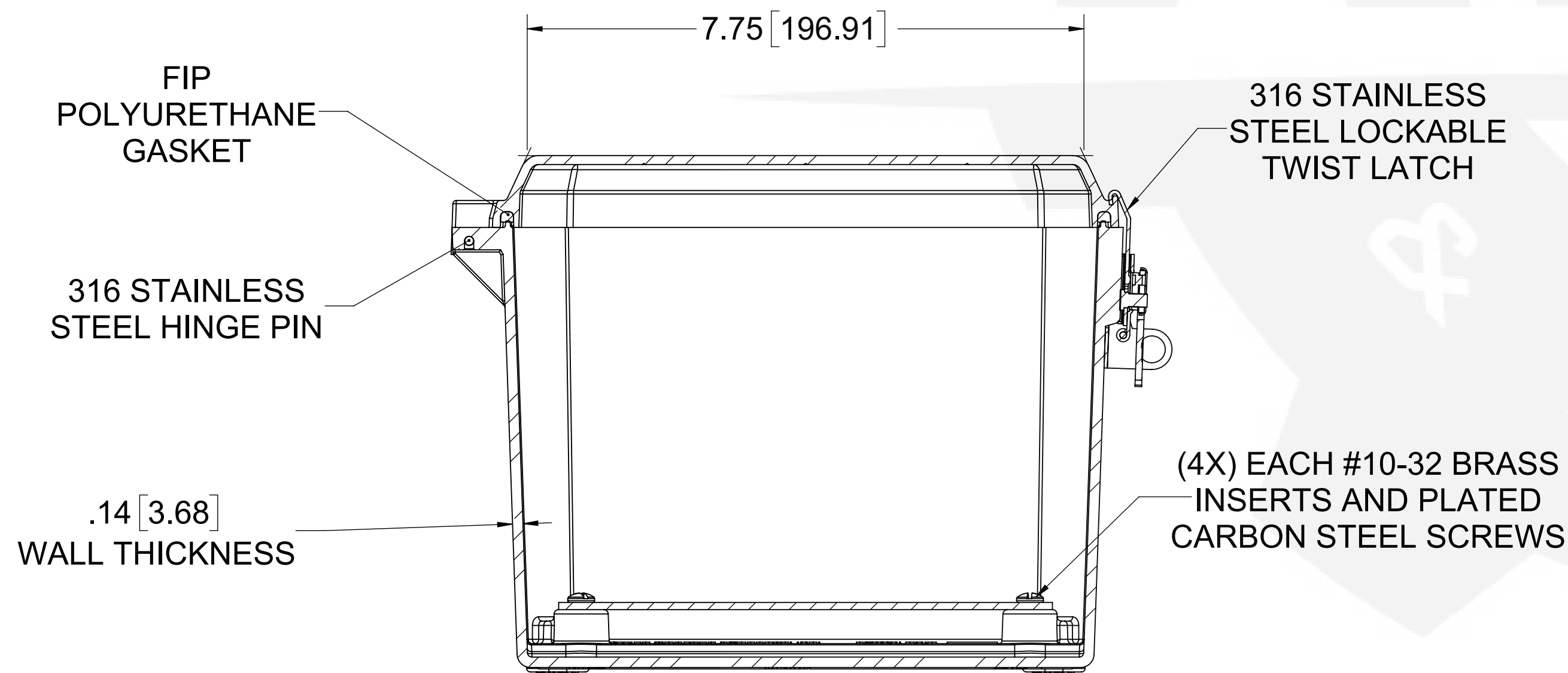
SECTION A-A
