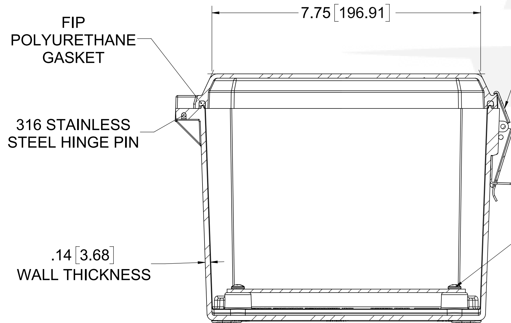
SECTION A-A
