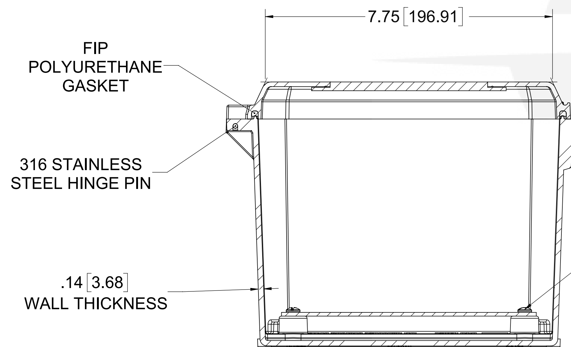
SECTION A-A
