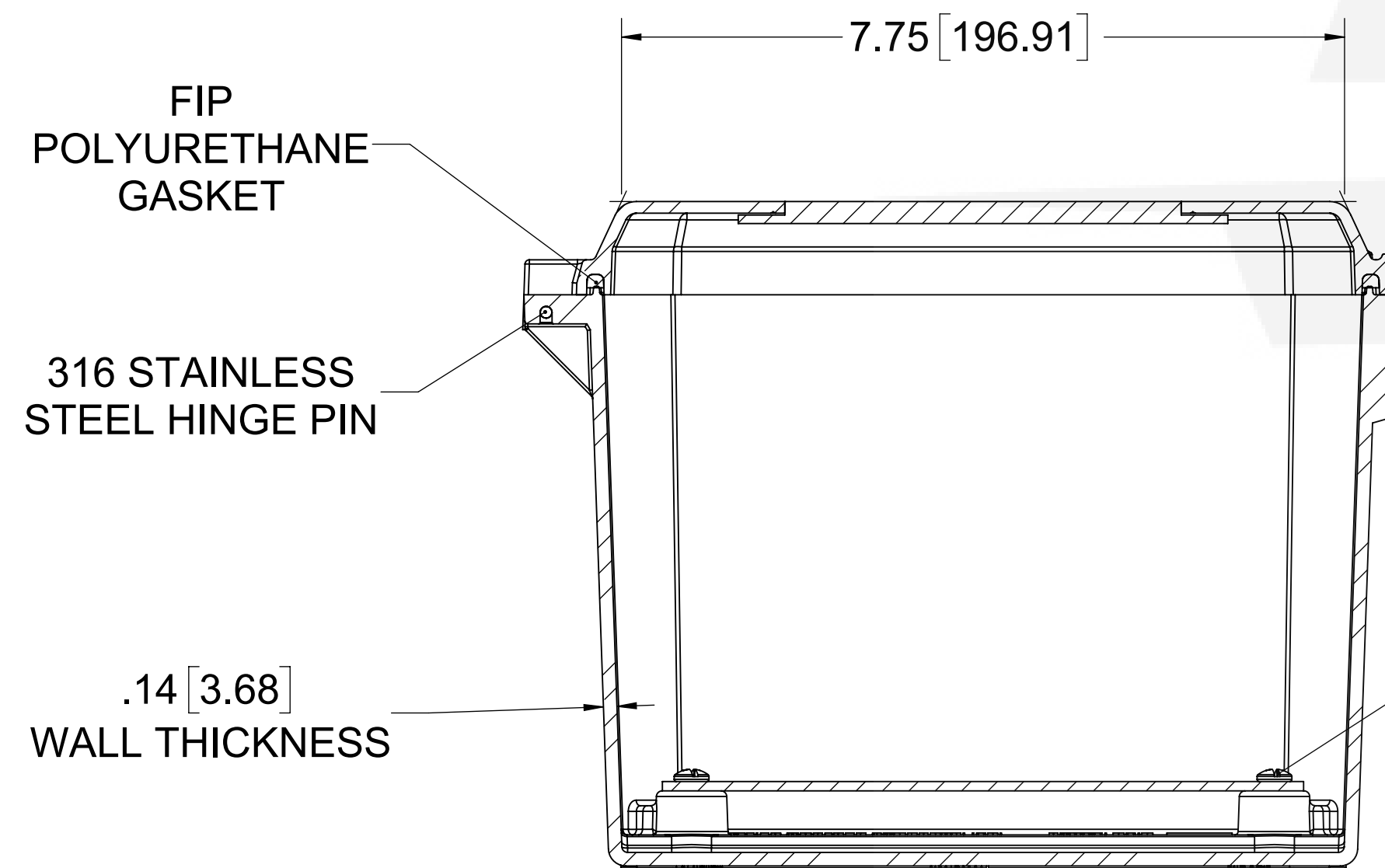
SECTION A-A
