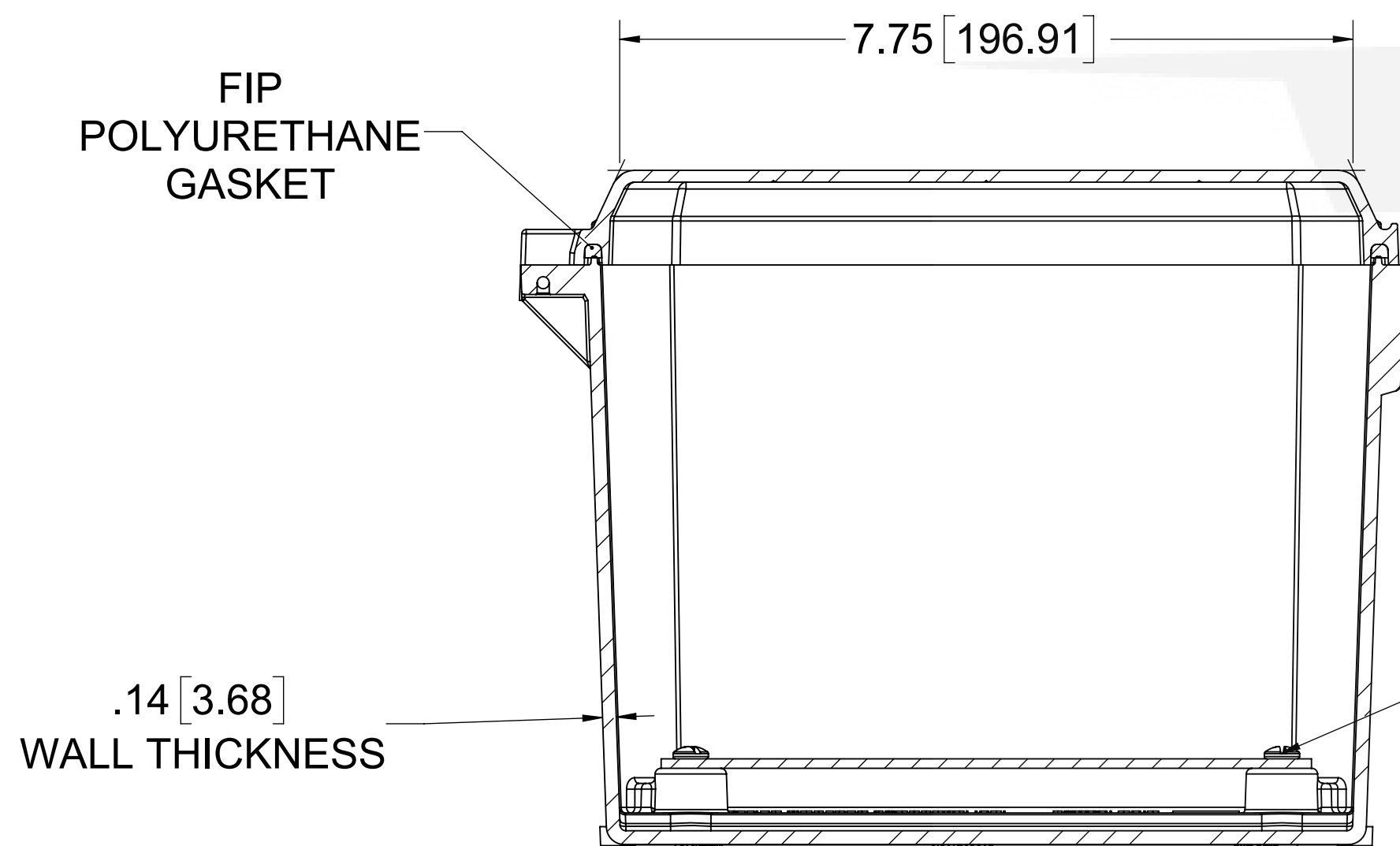
SECTION A-A
