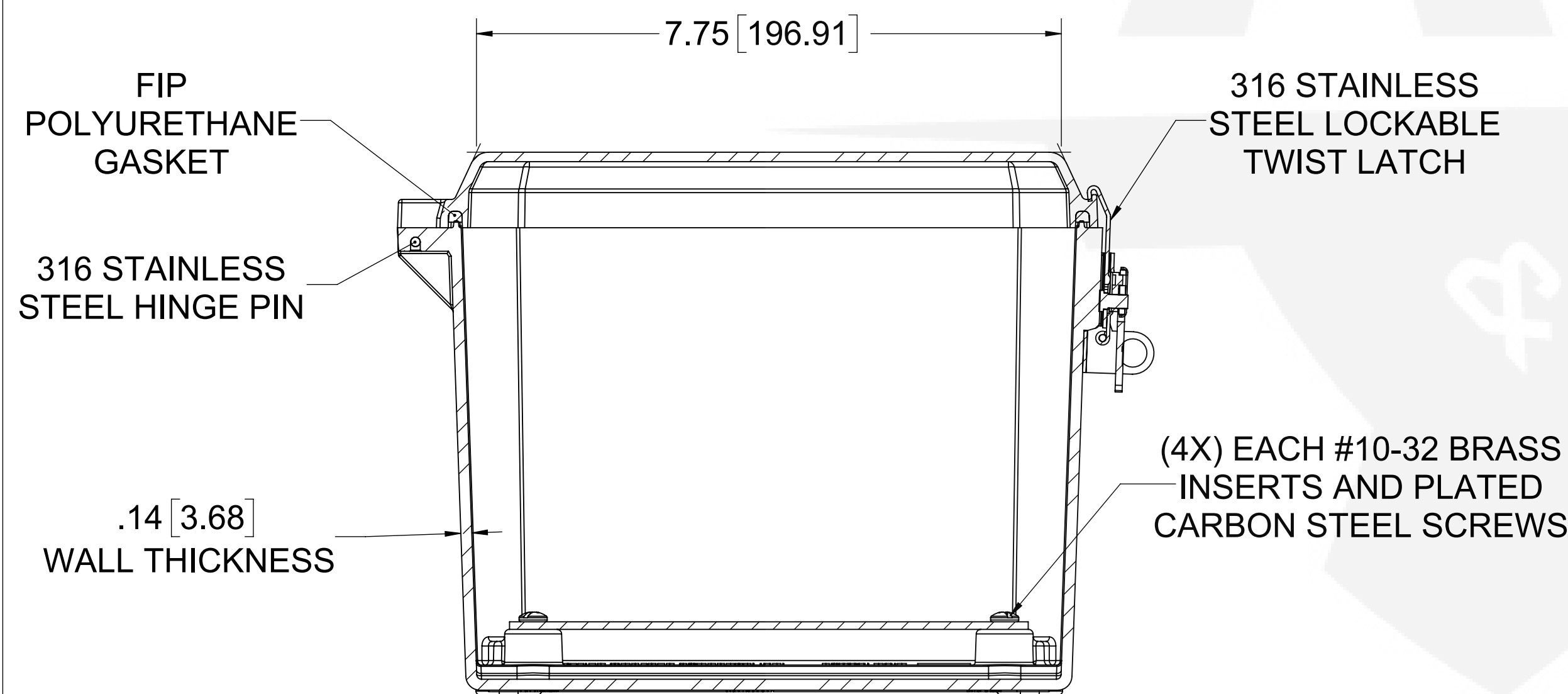
SECTION A-A
