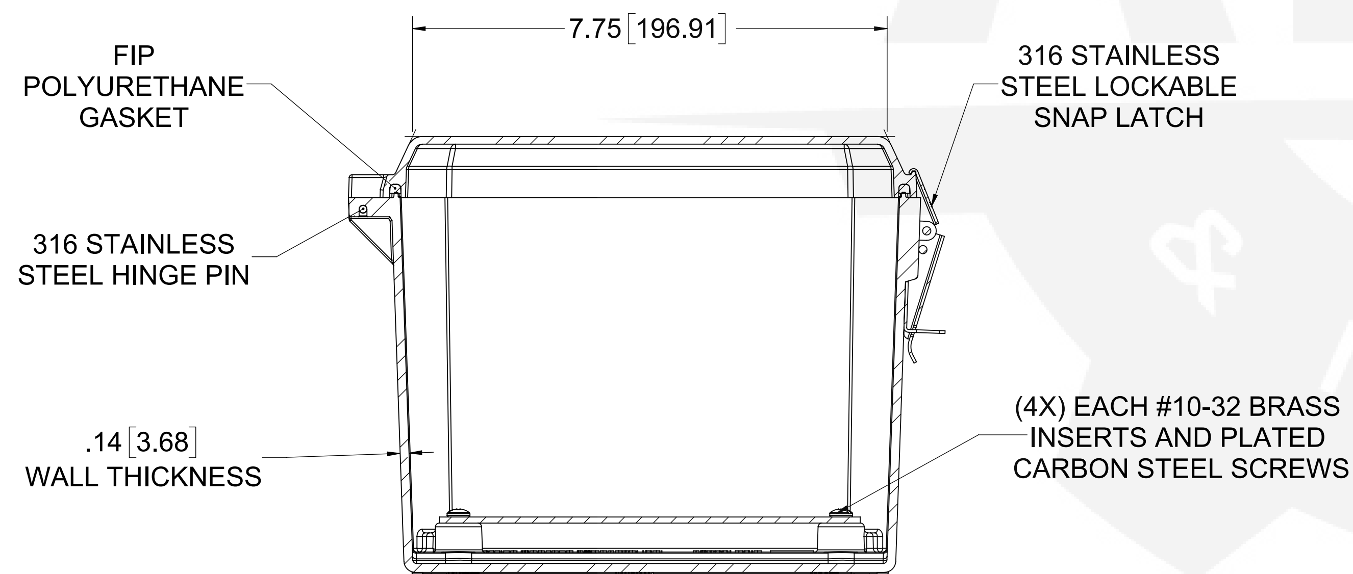
SECTION A-A
