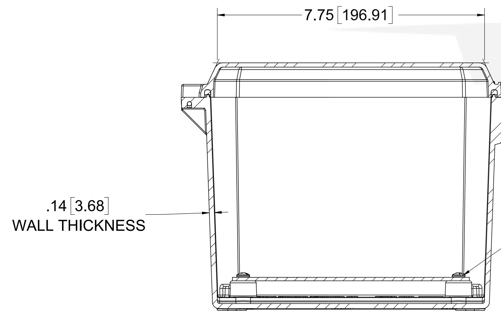
SECTION A-A
