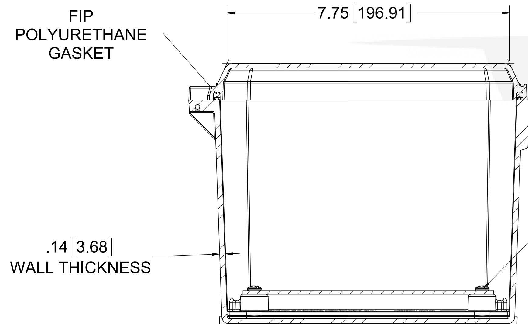
SECTION A-A
