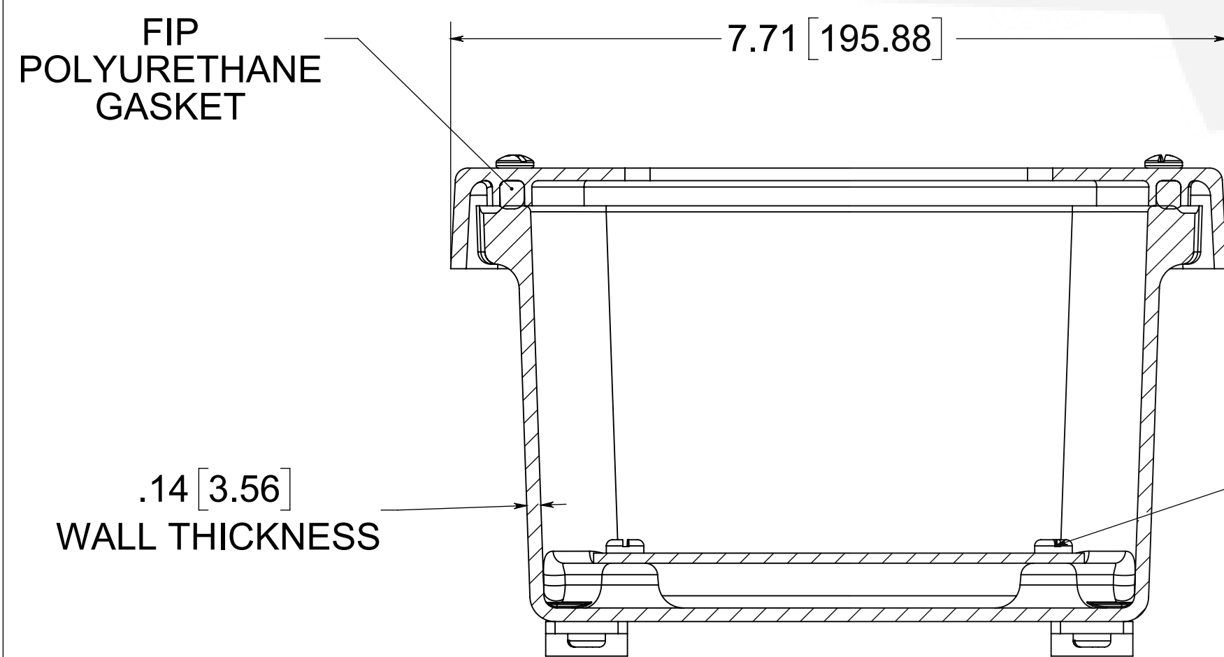
SECTION A-A
