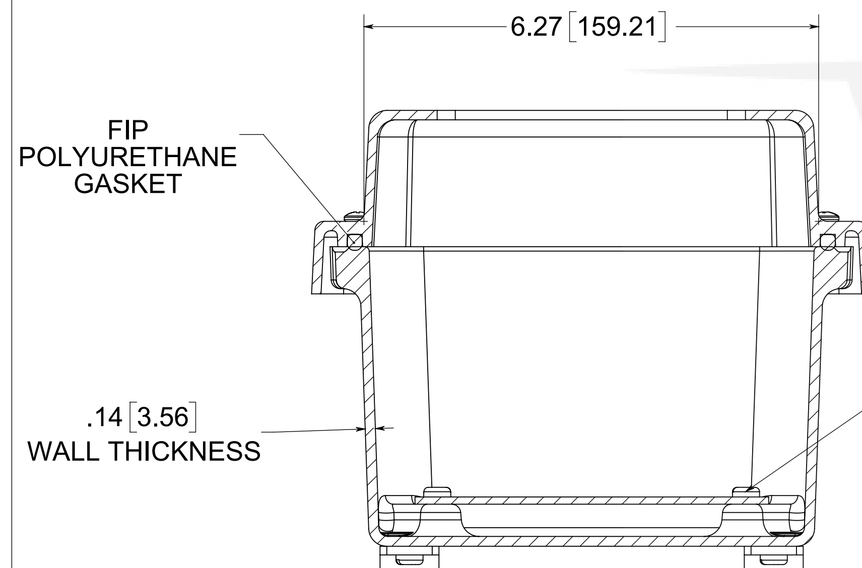
SECTION A-A
