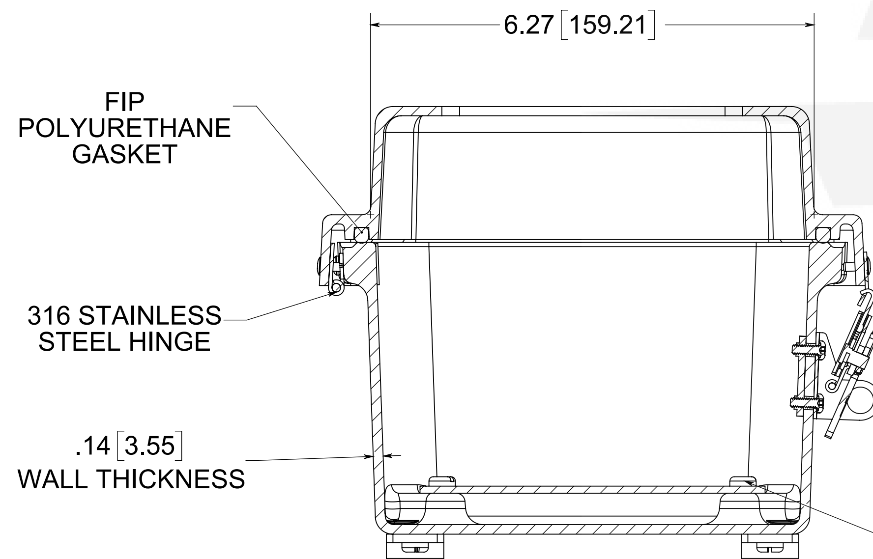
SECTION A-A
