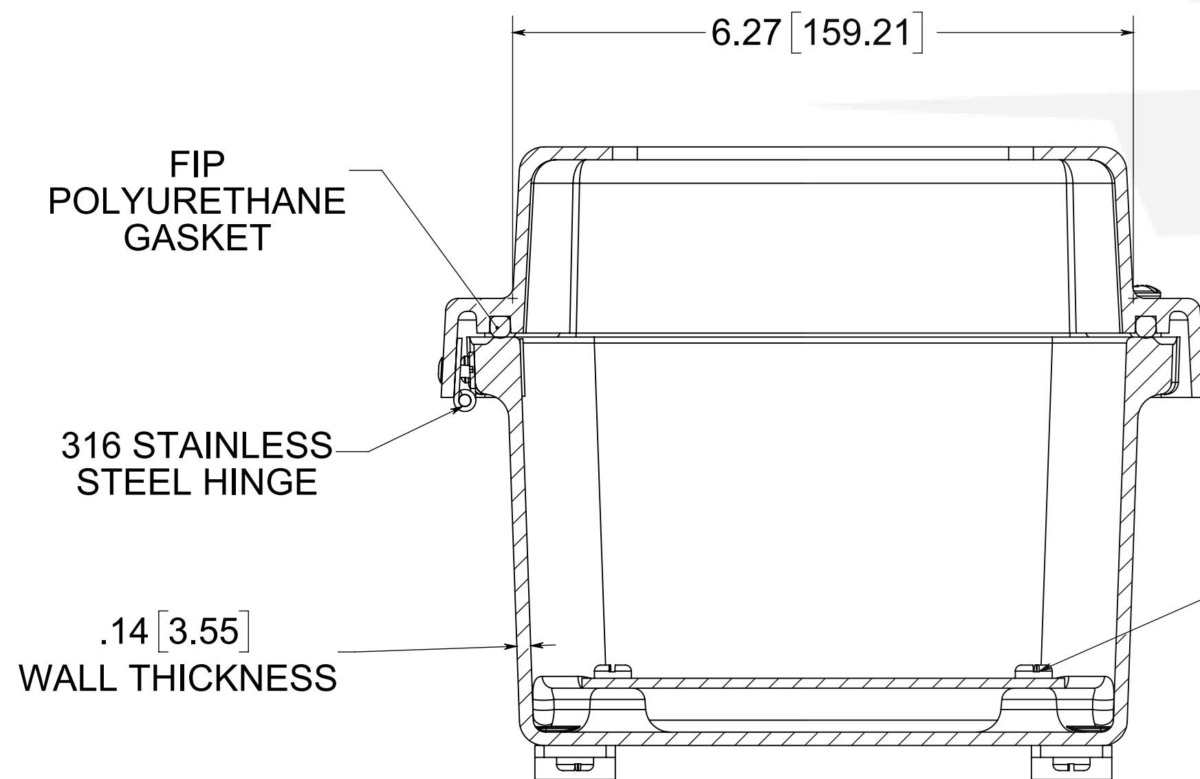
SECTION A-A
