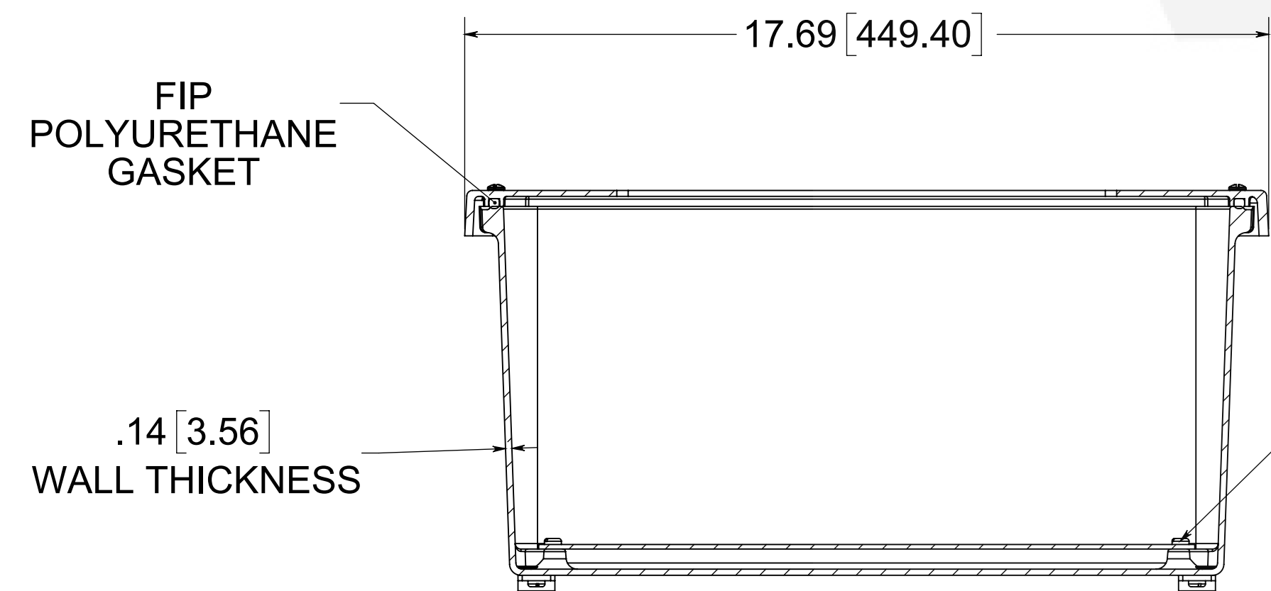
SECTION A-A
