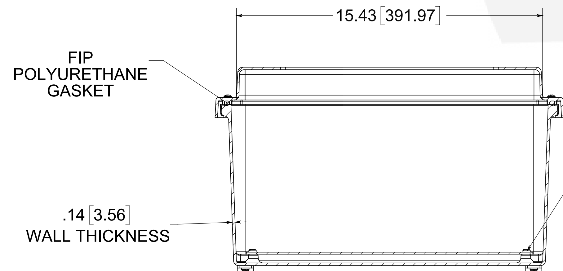
SECTION A-A
