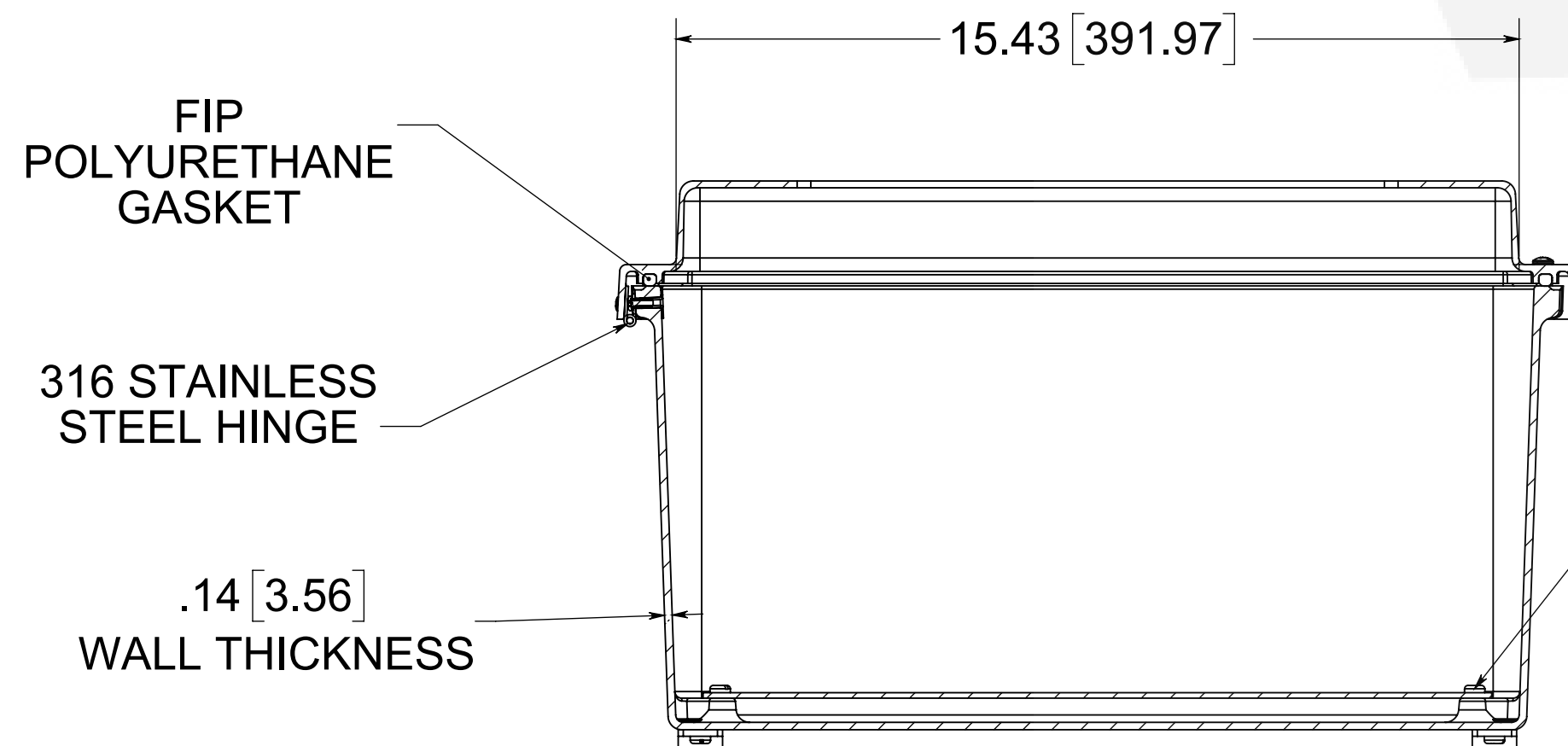
SECTION A-A
