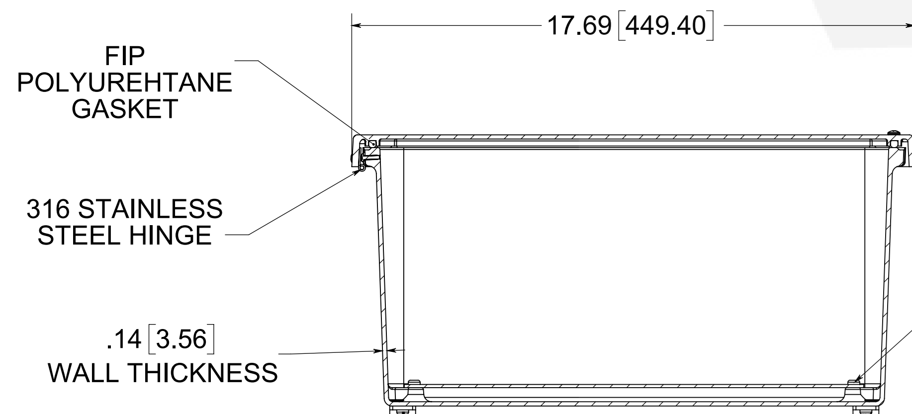
SECTION A-A
