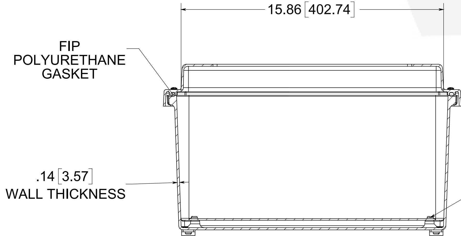
SECTION A-A
