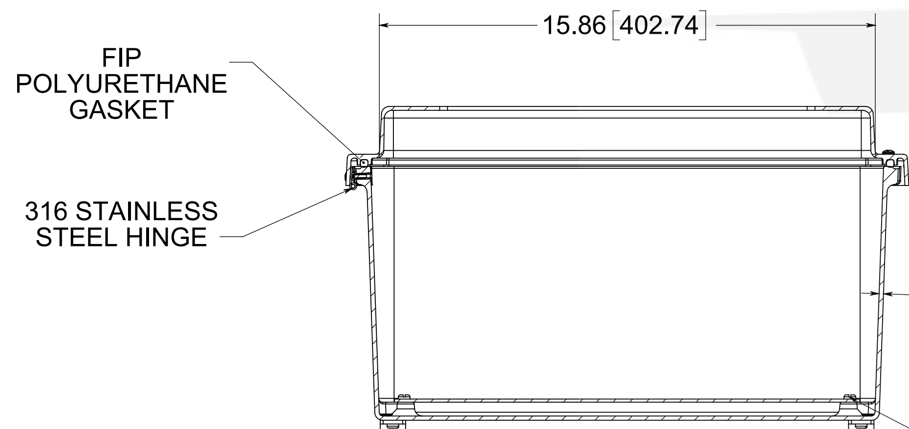
SECTION A-A
