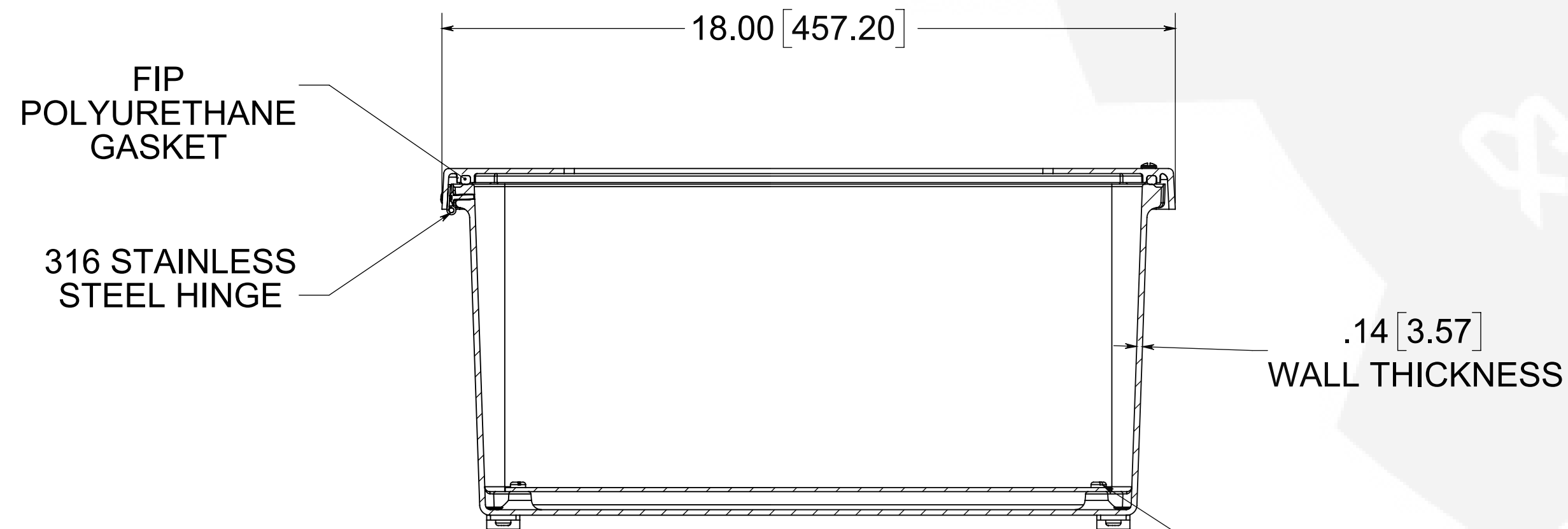
SECTION A-A
