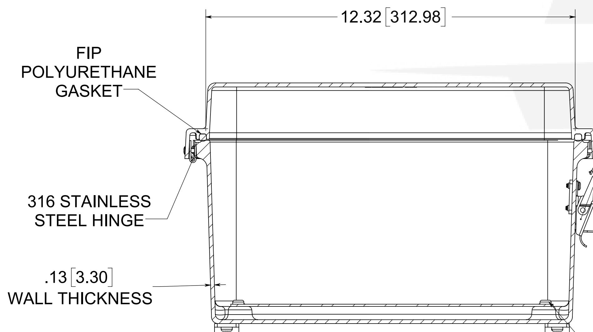
SECTION A-A
