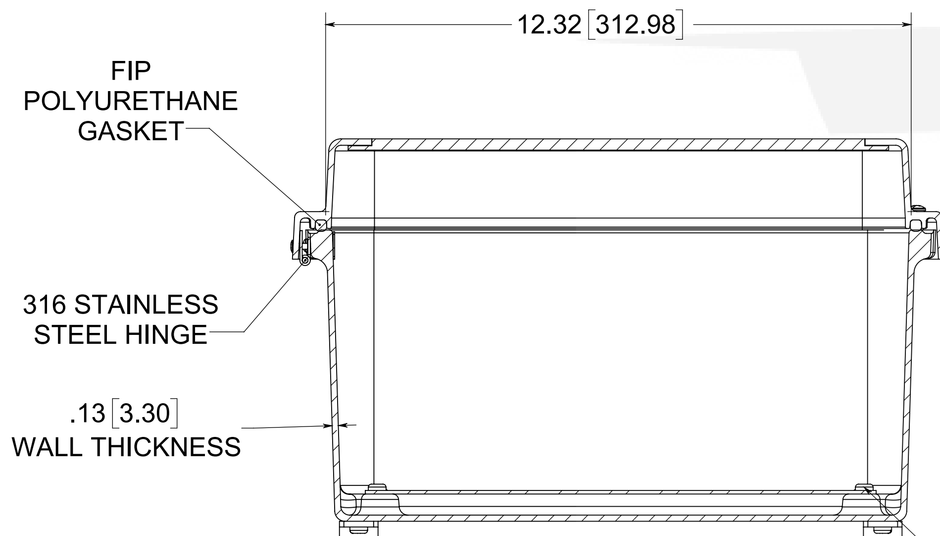
SECTION A-A
