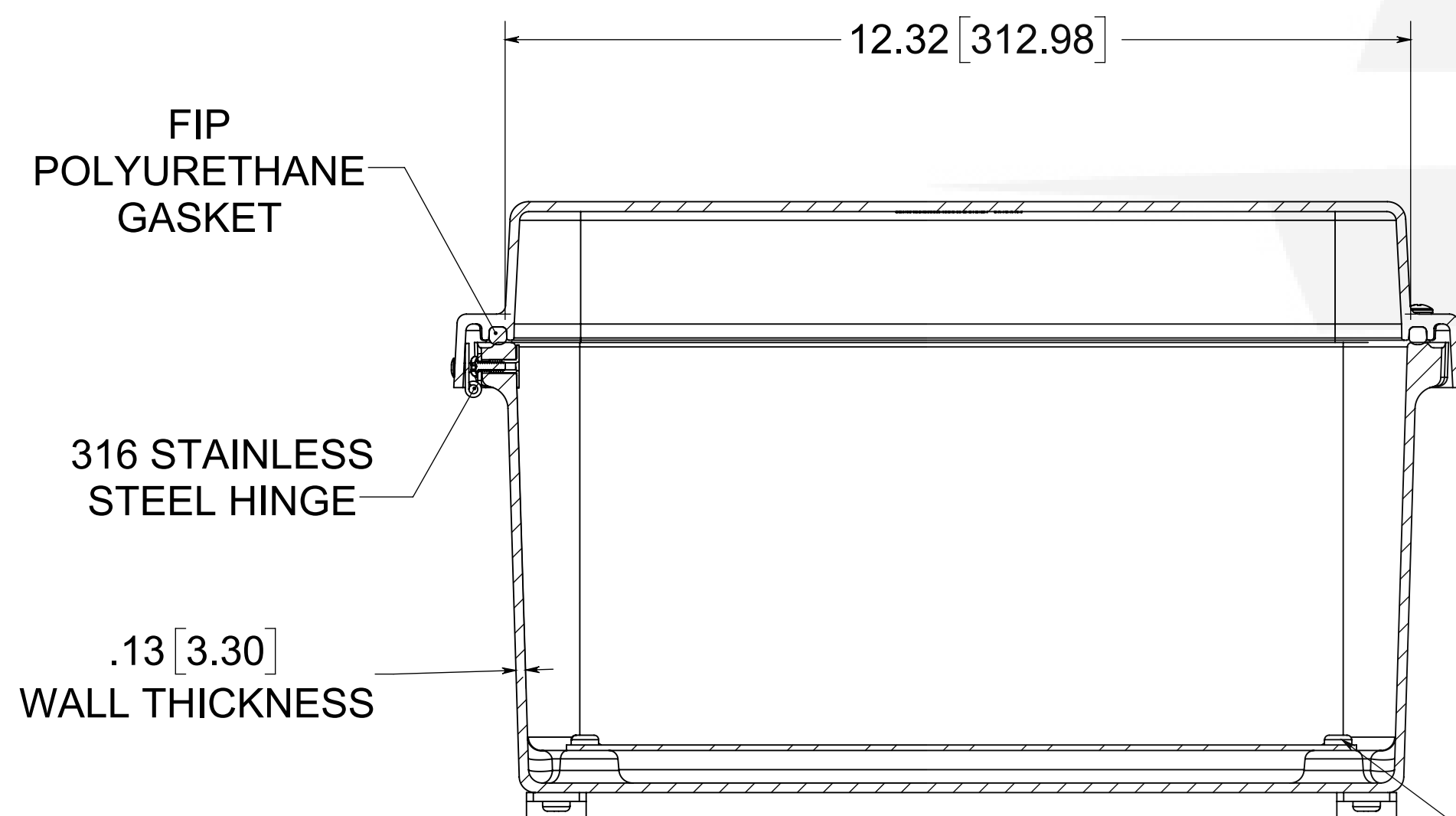
SECTION A-A
