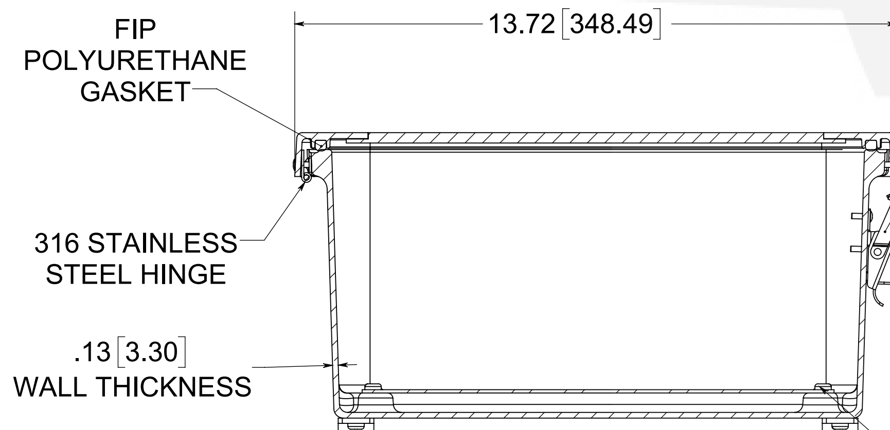
SECTION A-A
