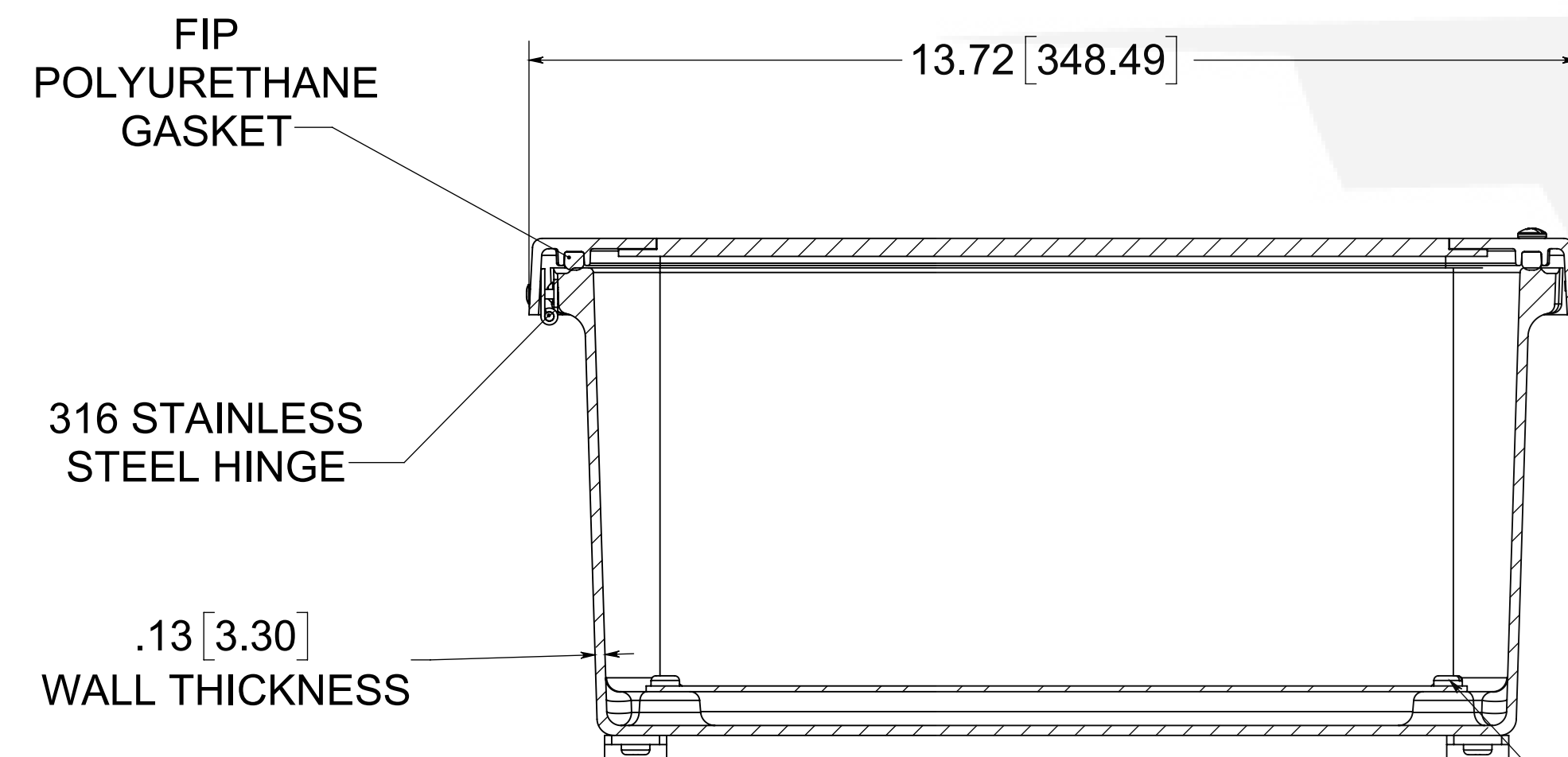
SECTION A-A
