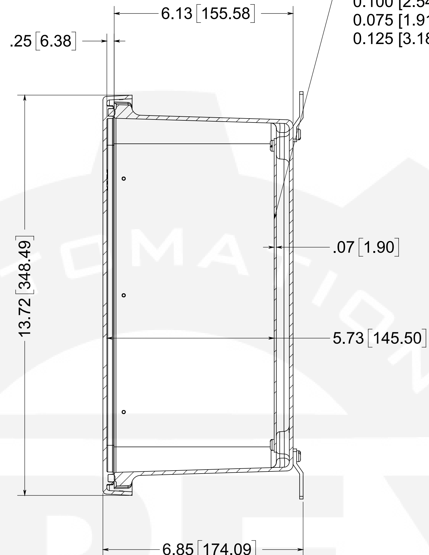
SECTION A-A
