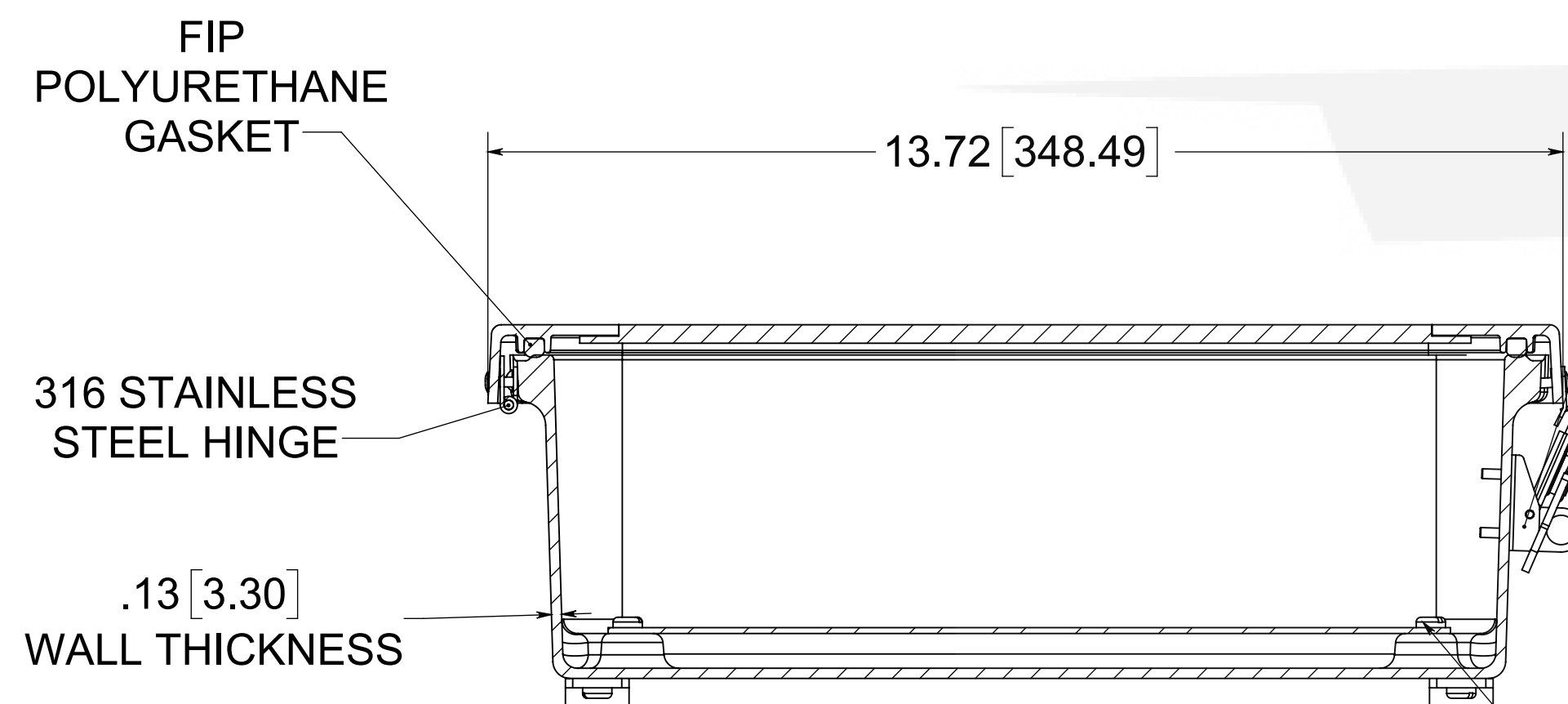
SECTION A-A
