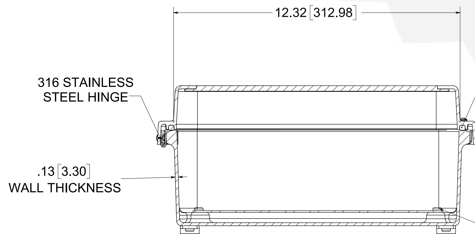
SECTION A-A
