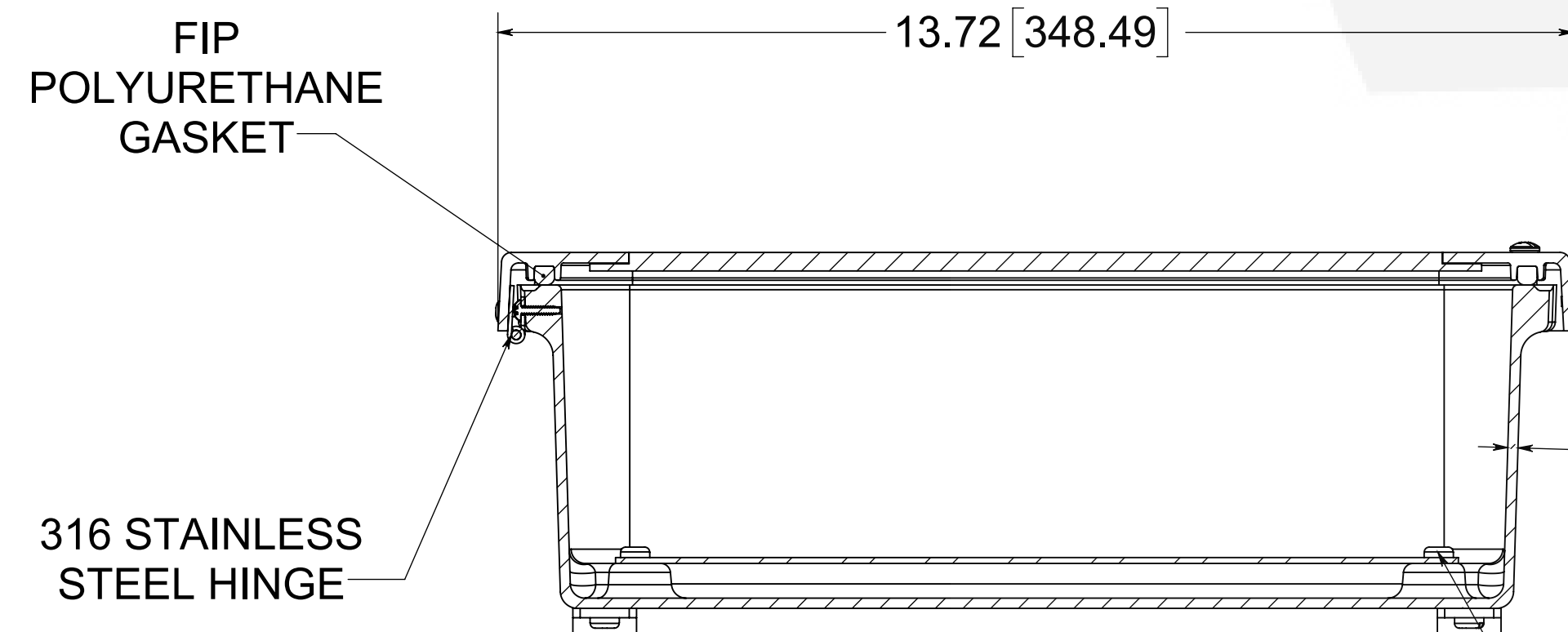
SECTION A-A
