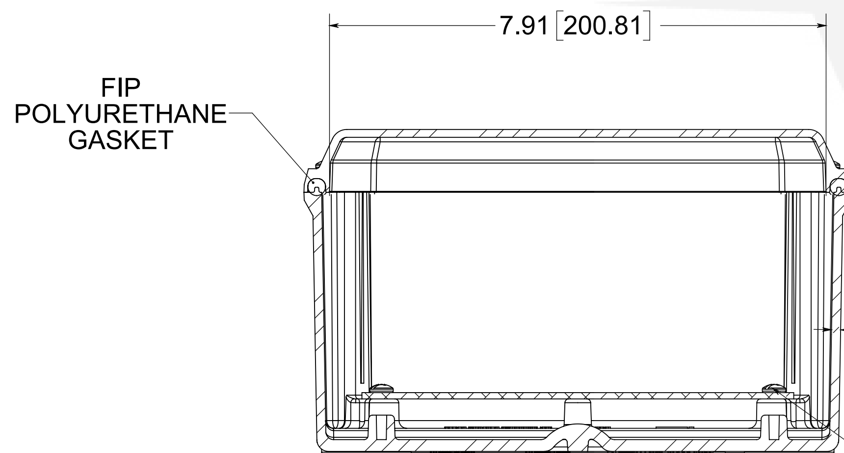
SECTION A-A
