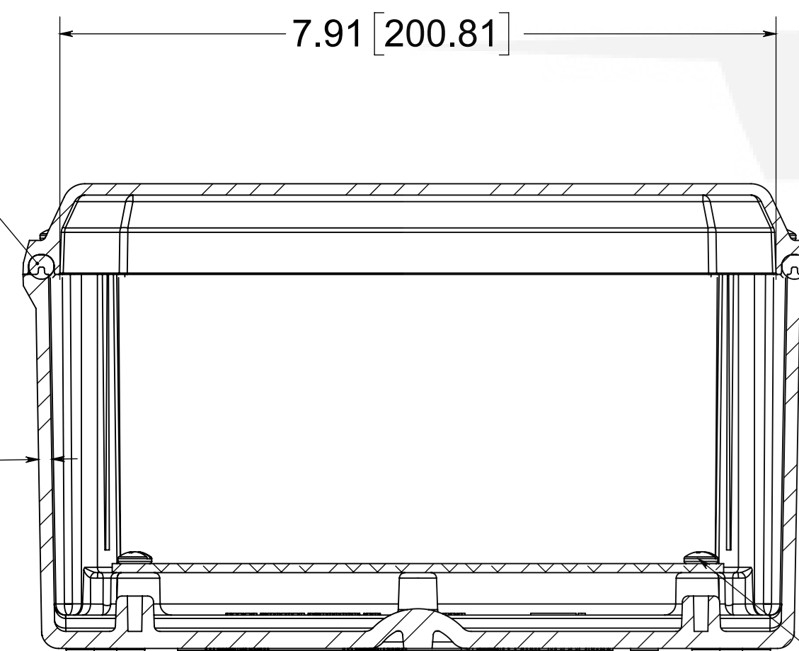
SECTION A-A
