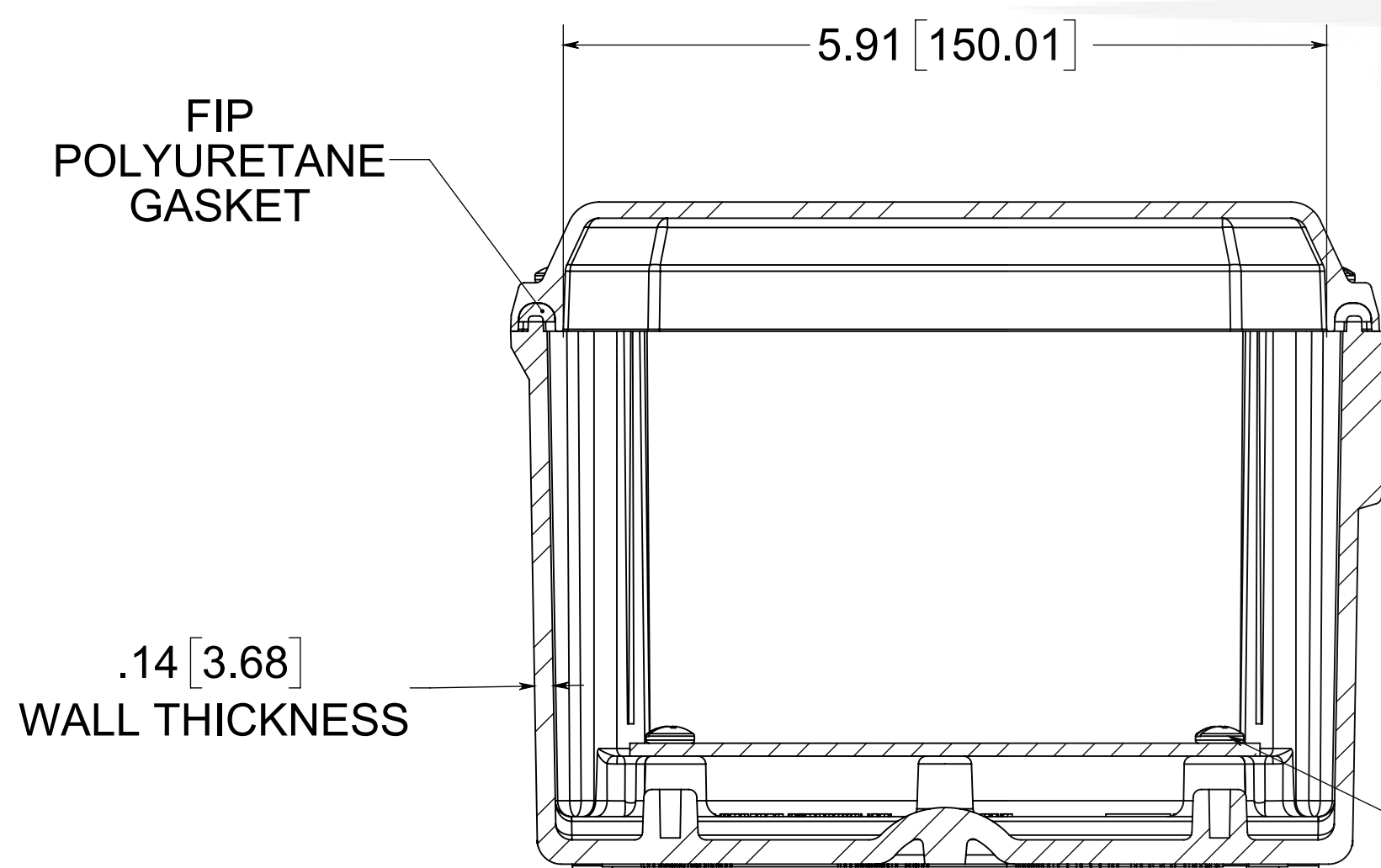
SECTION A-A
