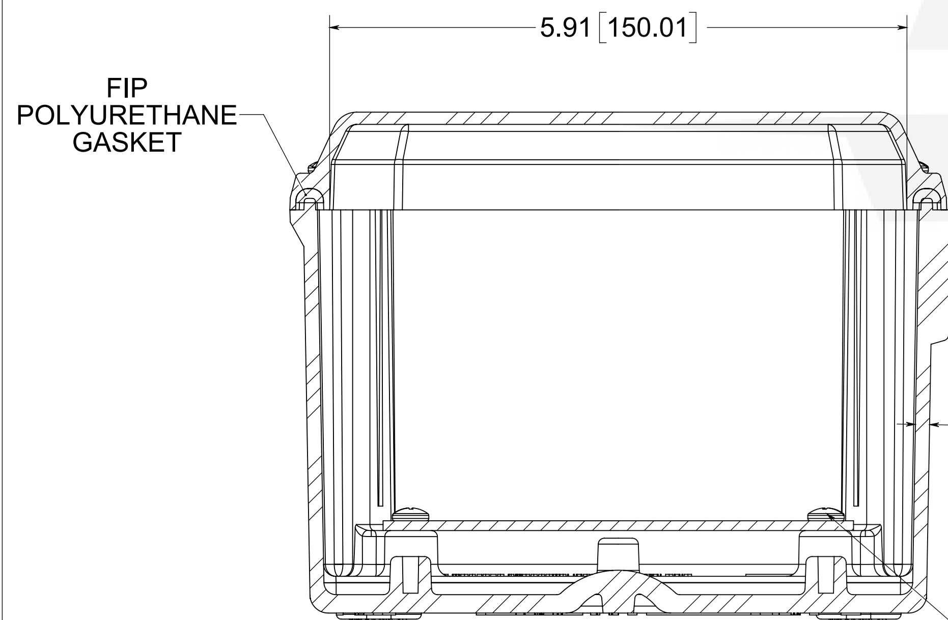
SECTION A-A
