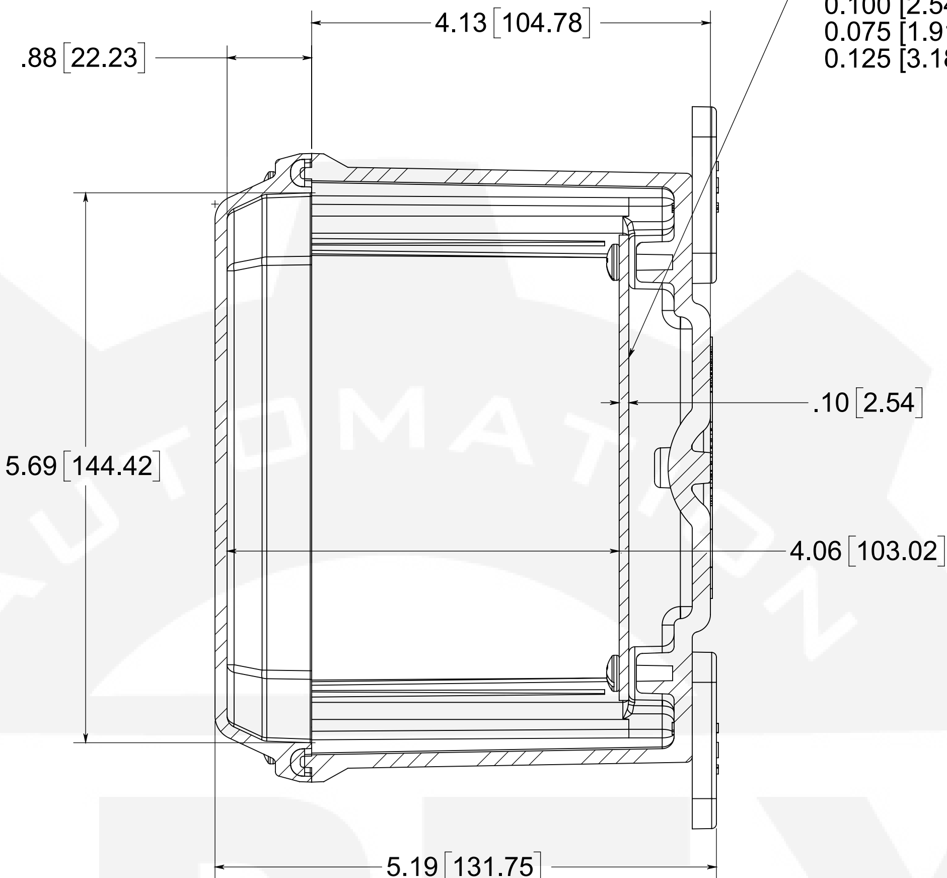
SECTION A-A
