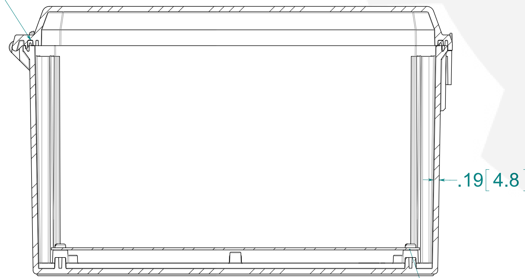
SECTION D-D
