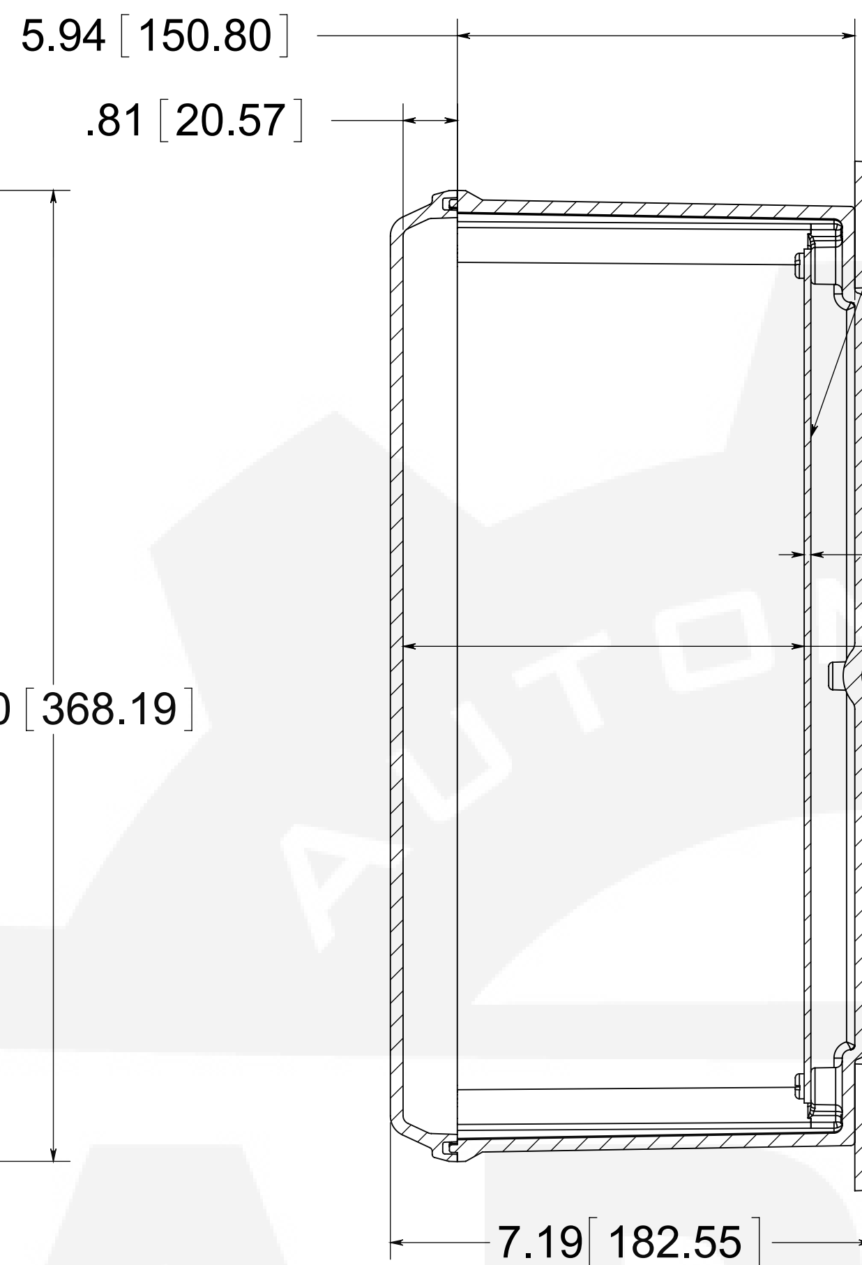
SECTION A-A
