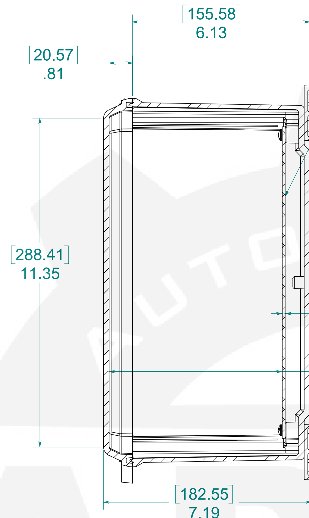
SECTION A-A
