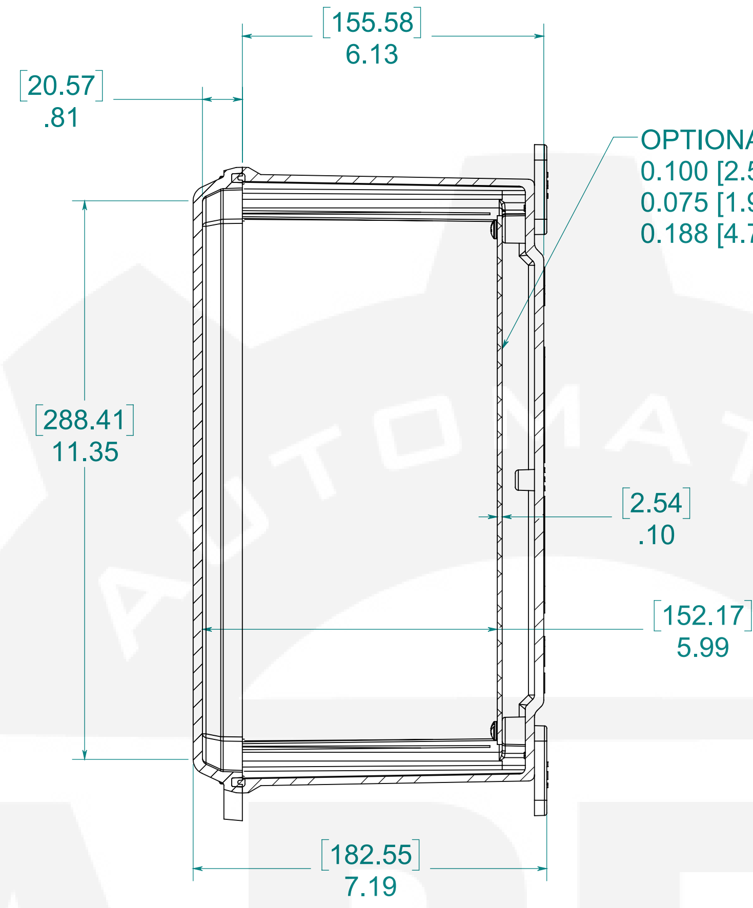
SECTION A-A
