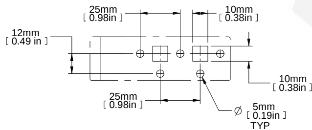
DETAIL A 10:1
