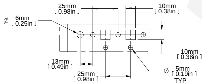
DETAIL A 10:1
