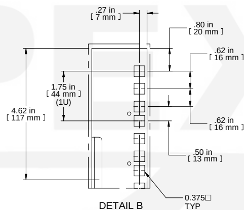
DETAIL B 5:1
