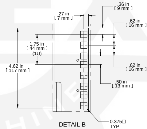
DETAIL B 5:1
