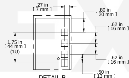
DETAIL B 5:1
