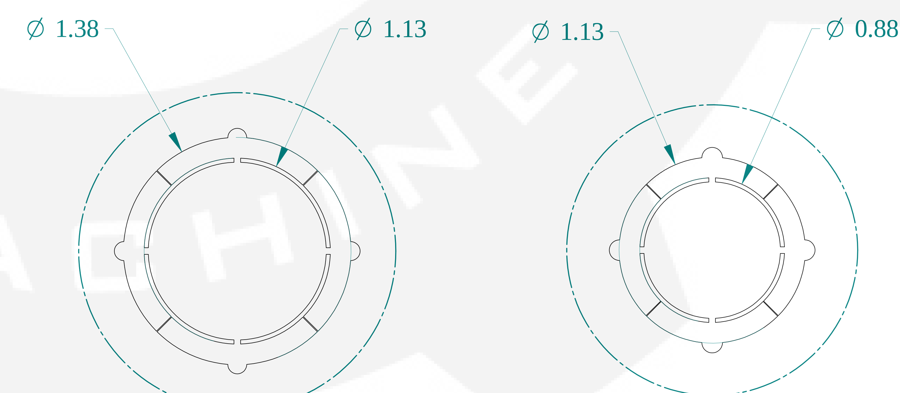
DETAIL Y TYP (10)
