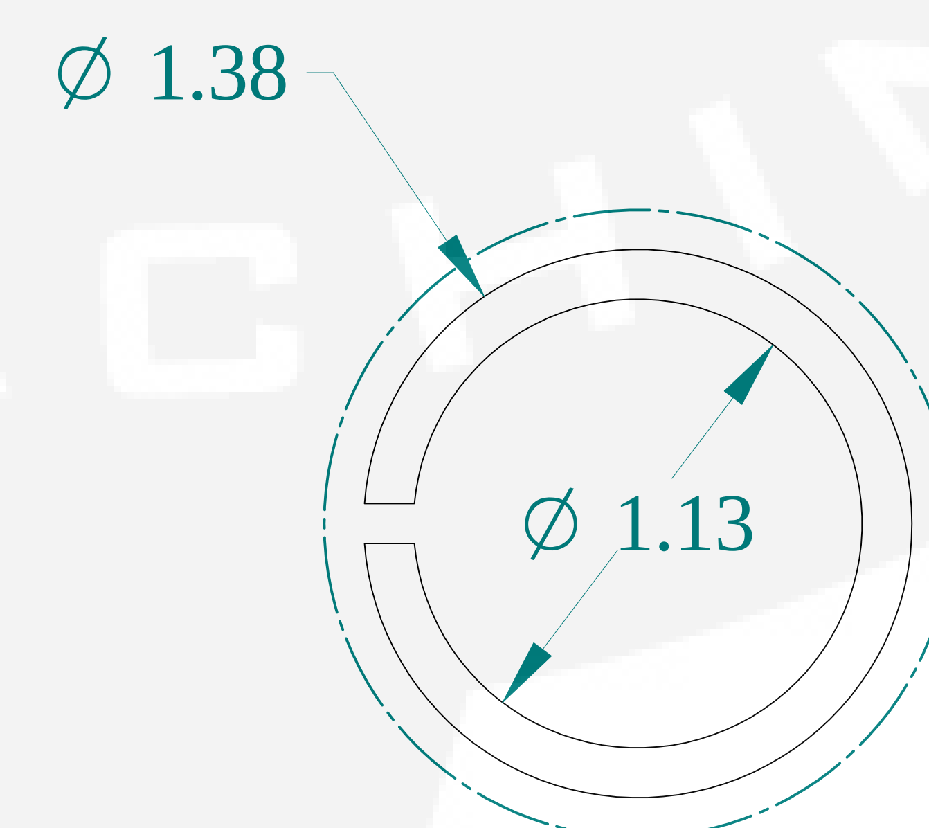
DETAIL Y
